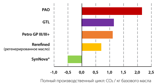
Выбросы CO 2 на всех этапах производства базовых масел (кг CO 2 / кг базового масла)
